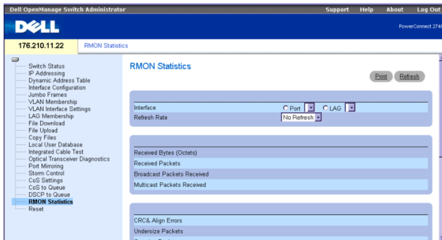
그림 8-1. RMON 통계
